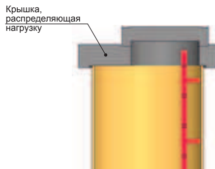
Рисунок 4-1-1-1 Типичное решение для крышек смотровых колодцев/камер, передающих нагрузку непосредственно
