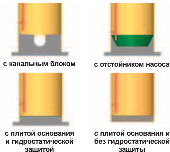
Рисунок 4-2-1 Виды оснований смотрового колодца
