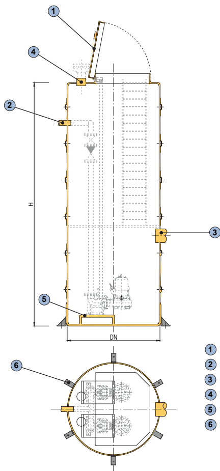
Рисунок 3-2-1 Возможное решение для размещения насосной станции в стеклопластиковом смотровом колодце в зонах без нагрузки транспорта, основанное на тонкостенной стеклопластиковой трубе, укрепленной ребрами
