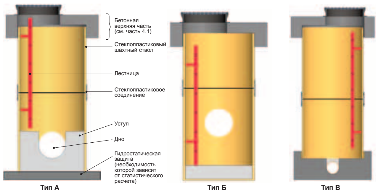
Рисунок 2-1-1 Цилиндрические стеклопластиковые смотровые колодцы типа А, Б, и В
