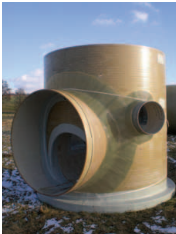
Рисунок 2-6-1 Стеклопластиковый смотровой колодец для двойной трубной системы, используемой в защищенных зонах
