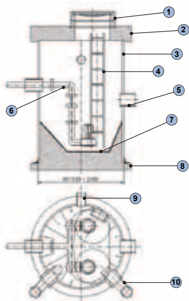
Рисунок 3-2-2 Возможное решение для размещения насосной станции в стеклопластиковом смотровом колодце, основанное на обычной стеклопластиковой трубе
