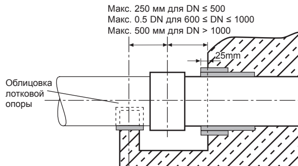
Рисунок 6-4 Вариант В: Резиновые прокладки
