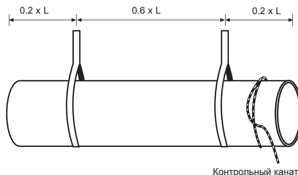
Рисунок 2-2 Подъем трубы с использованием двух точек опоры
