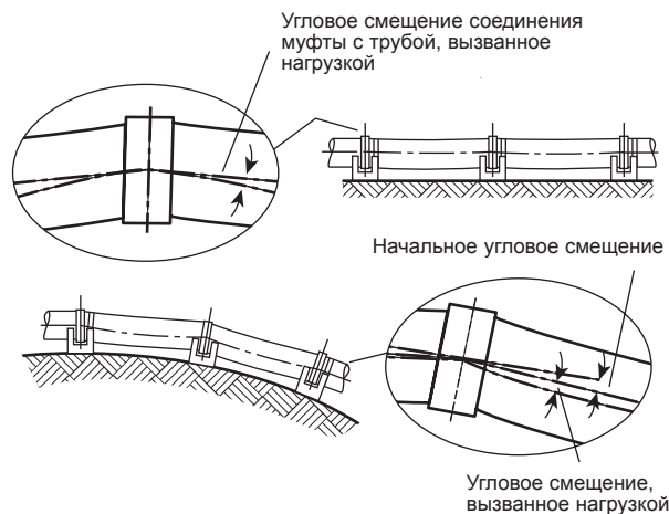
Рисунок 3-7 Смещение трубы
