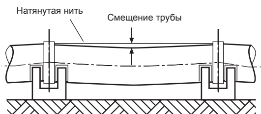
Рисунок 5-2 Смещение трубы
